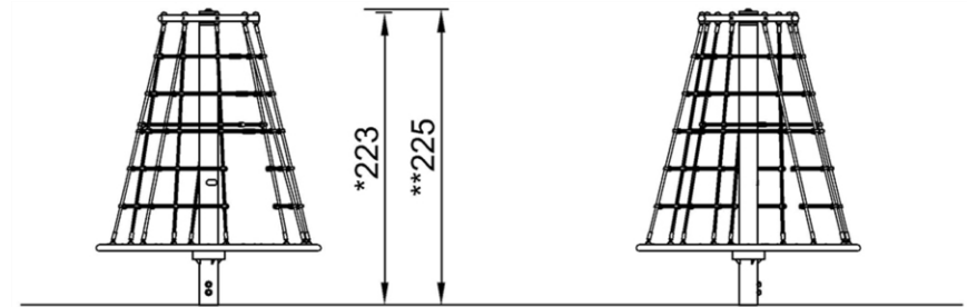
COR203301 1:100
